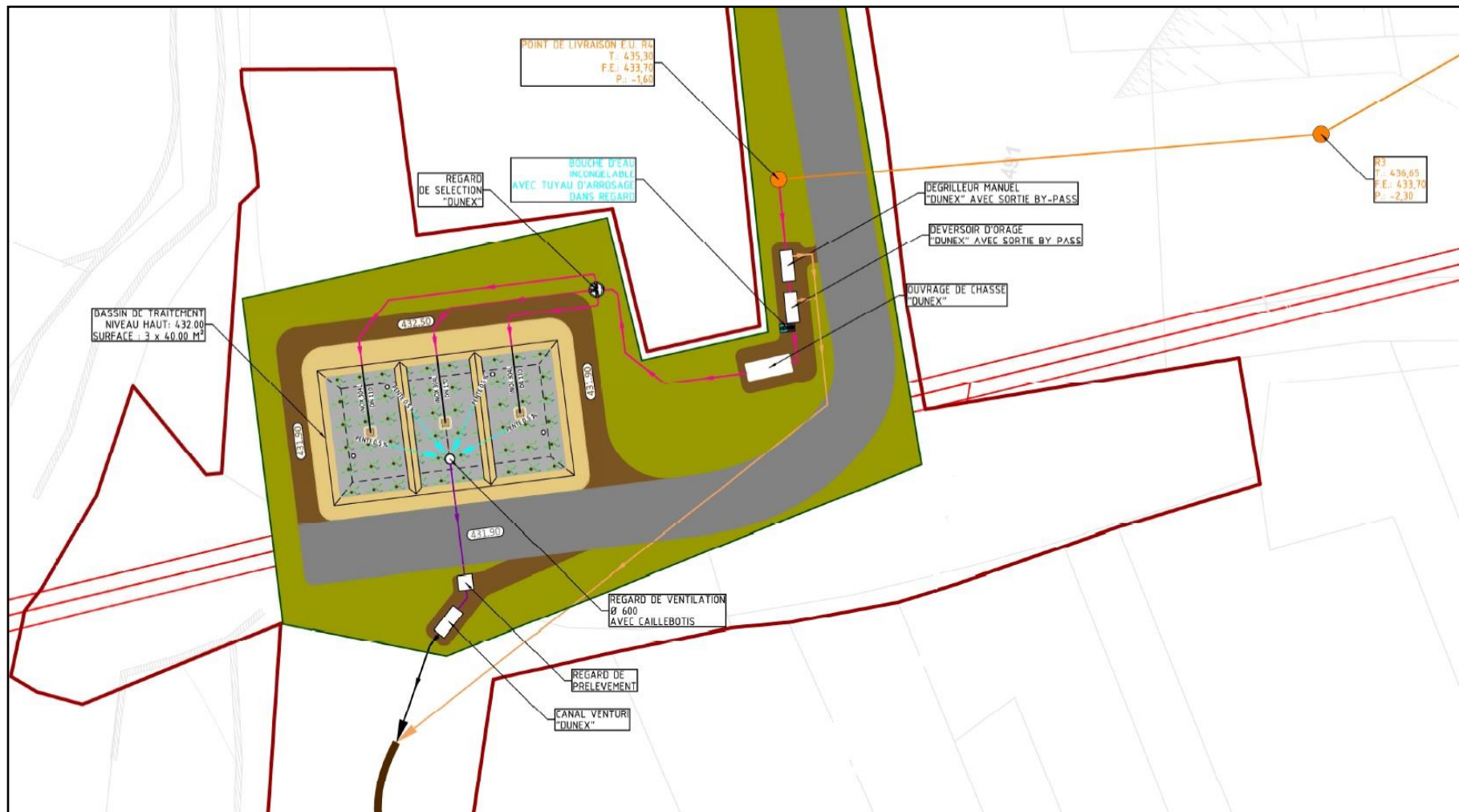
Plan de la STEP de Mont de l'Ange
